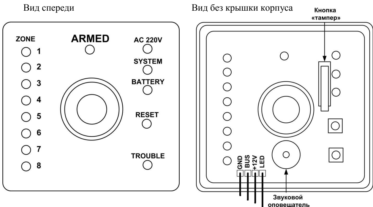
Рисунок 7. УИУ «Линд-11ТМ»
