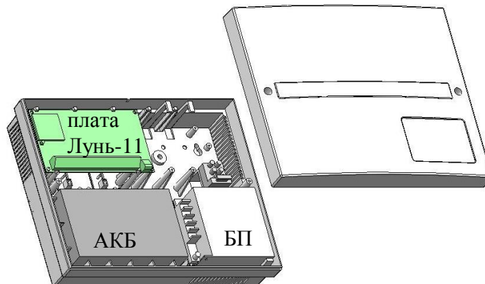
Рисунок 2. ППКОП «Лунь-11» (крышка снята)
