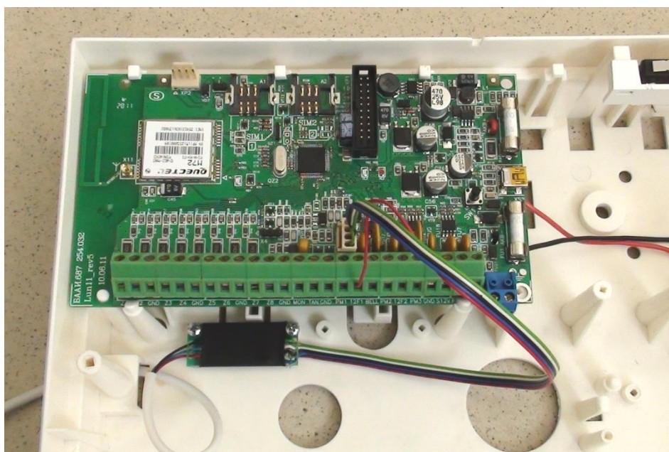
Рис. 9. Пример закрепления платы адаптера «Астра-Лунь-11»
