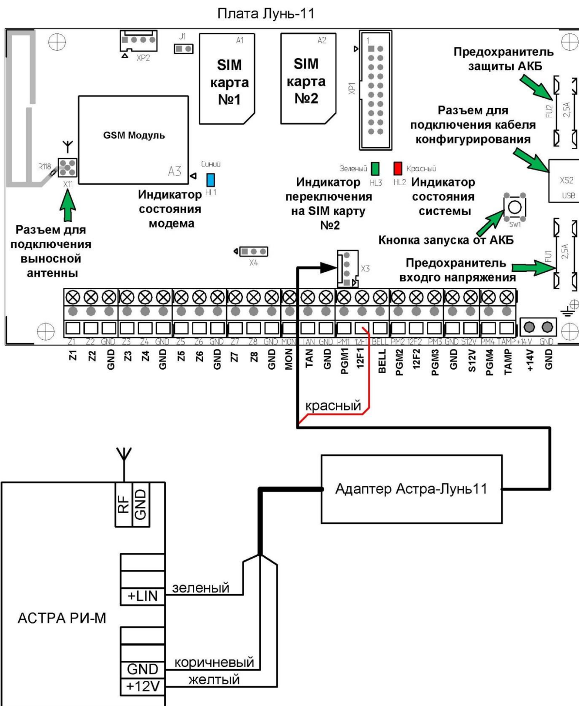
Рисунок 10. Схема подключения «РПУ Астра-РИ-М» к ППК «Лунь-11»
