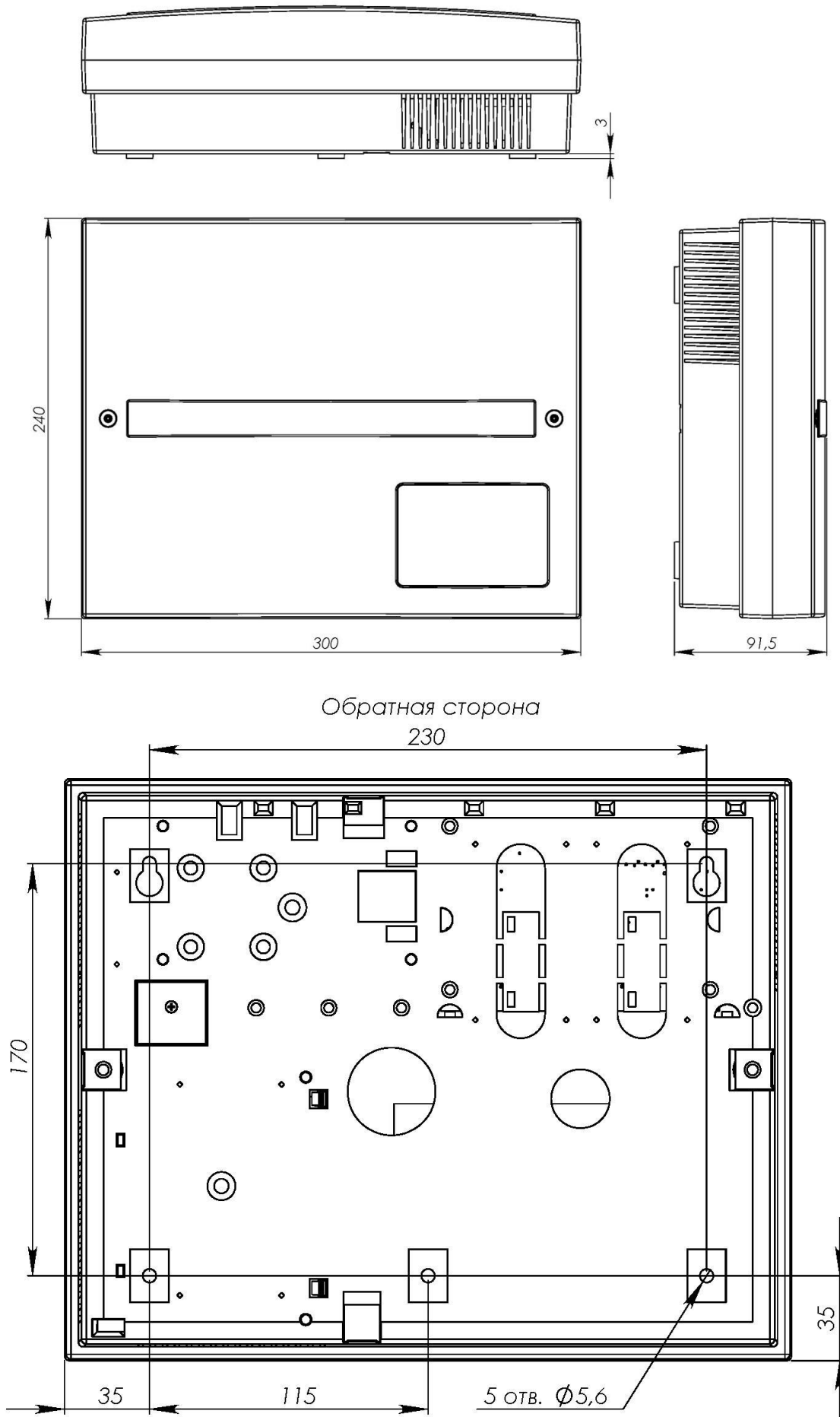
Рисунок 3. Габаритные и установочные размеры.
