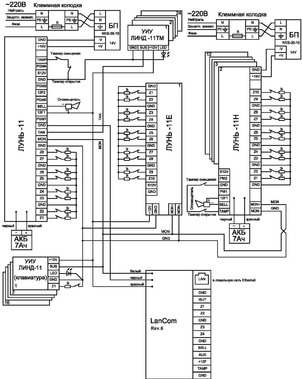
Рисунок 14. Схема подключения сетевых устройств. Вариант 2. LanCom rev6.
