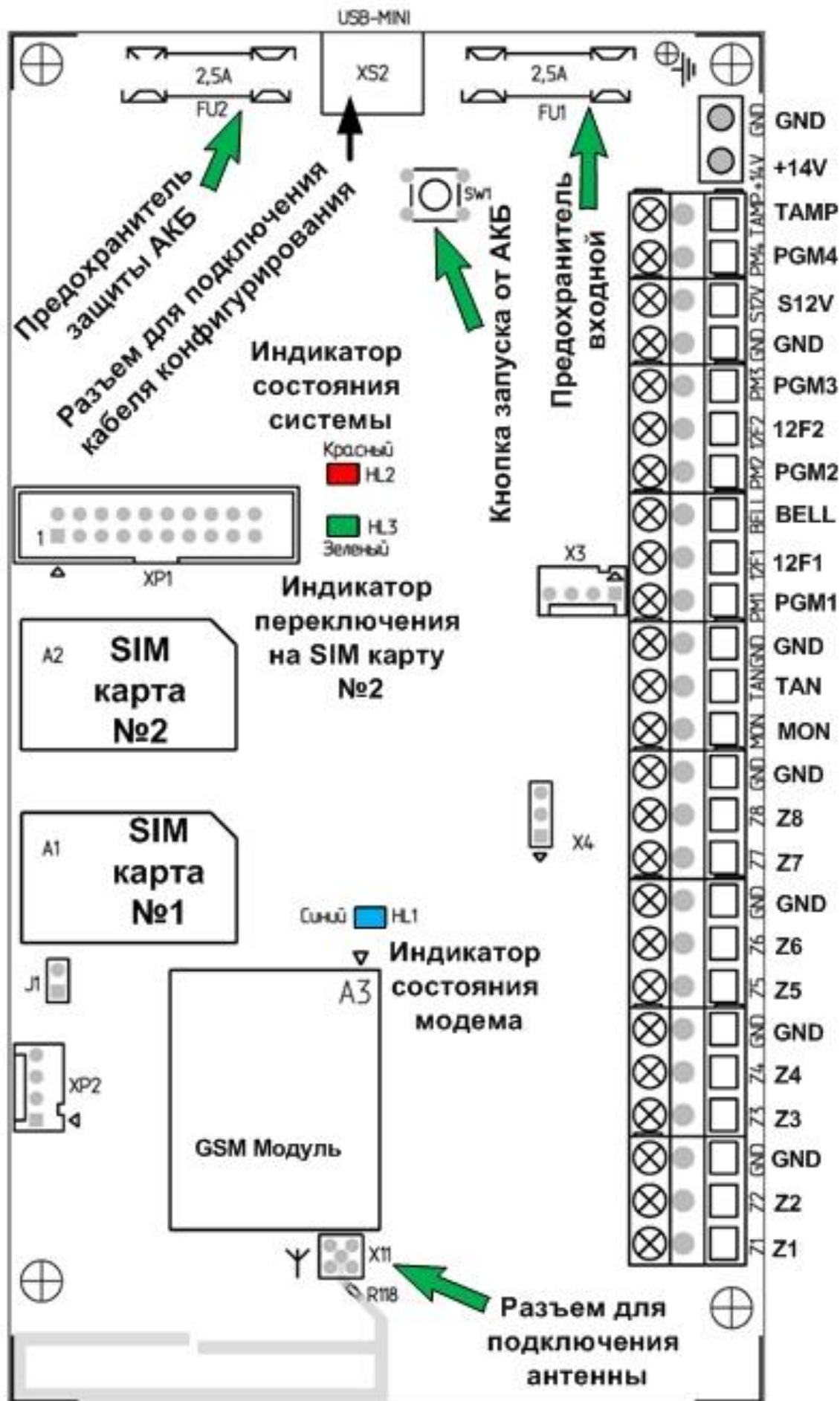
Рисунок 4. Внешний вид платы «Лунь-11».
