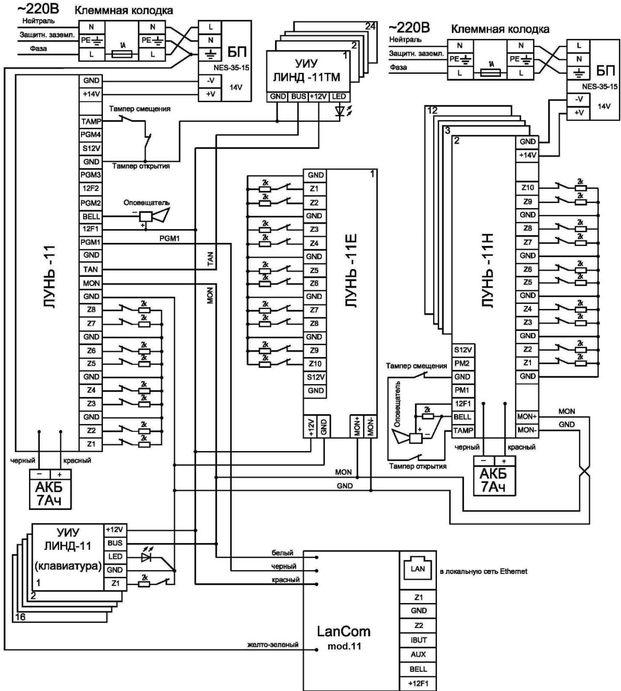
Рисунок 13. Схема подключения сетевых устройств. Вариант 1. LanCom mod11.
