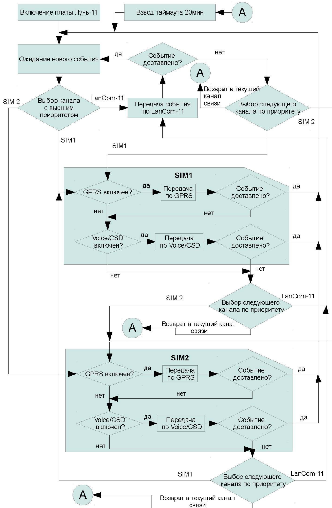
Рис. 6. Алгоритм выбора каналов передачи.
