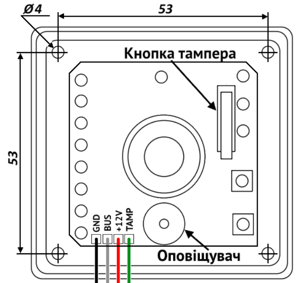
Малюнок 2. ПІК без верхньої кришки
