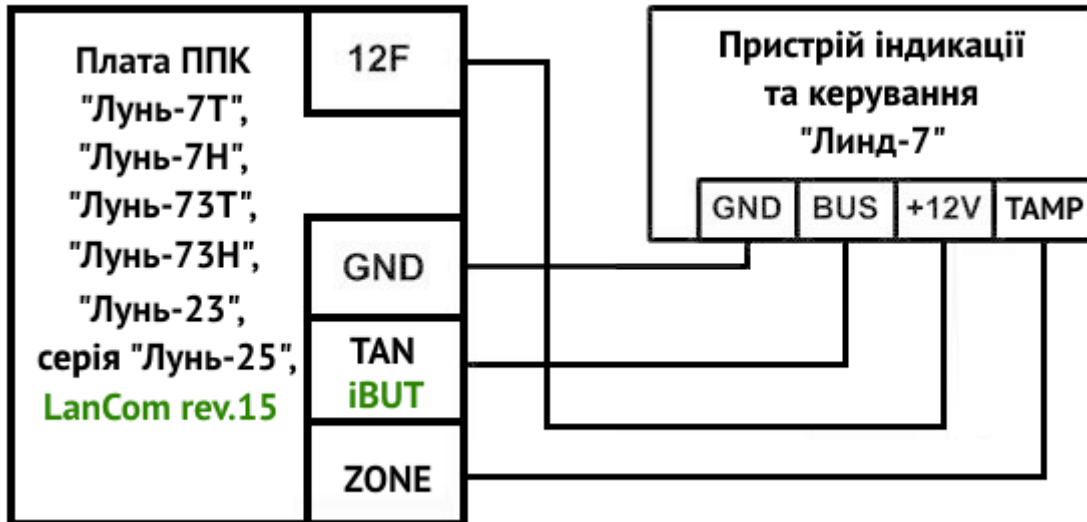
Малюнок 3. Схема під'єднання ПІК до ППК
