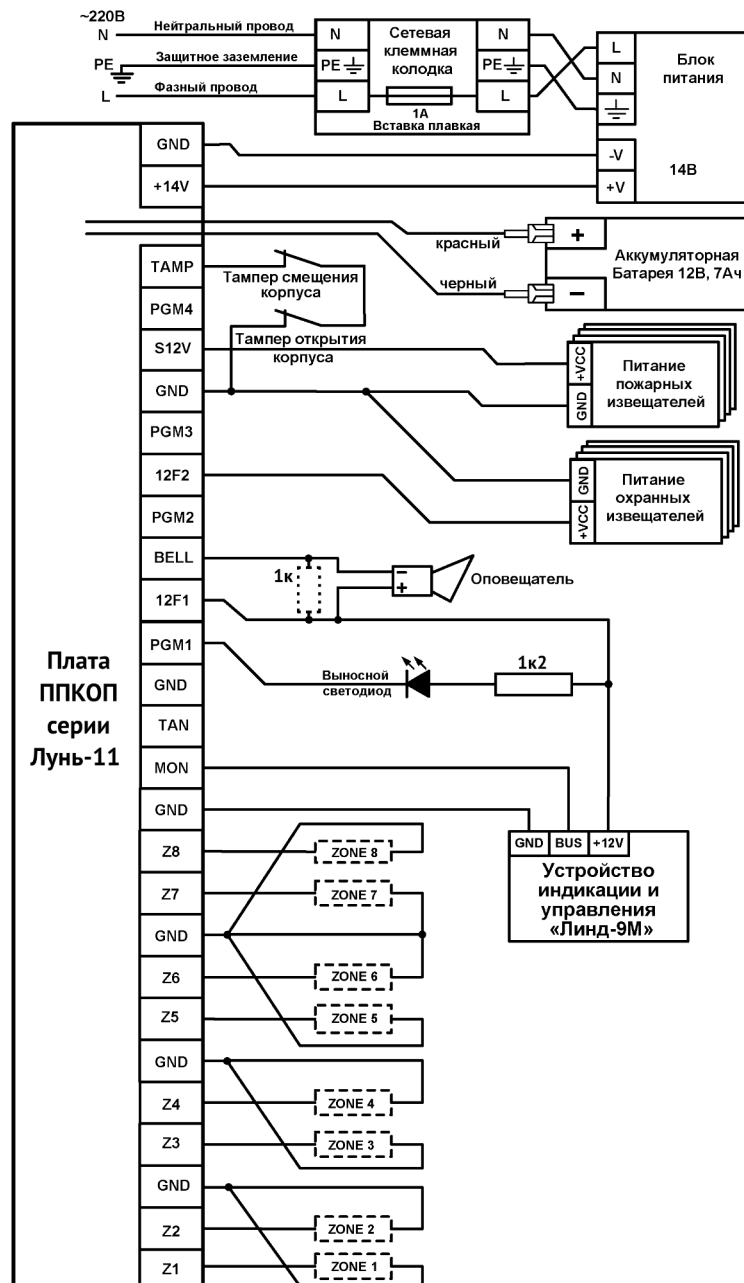
Рисунок 2. Схема подключения УИУ «Линд-9М»
