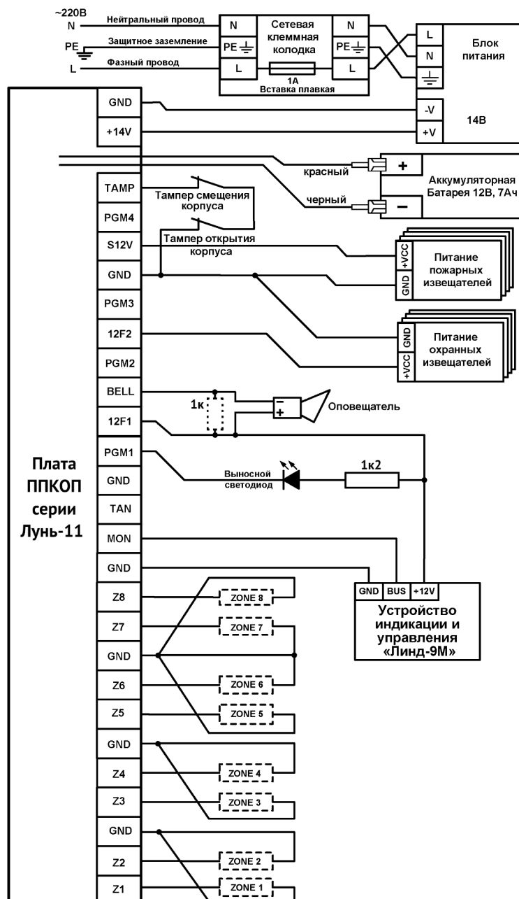
Рисунок 2. Схема подключения УИУ
