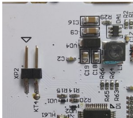
Рисунок 4. Разъем для обновления ПО
