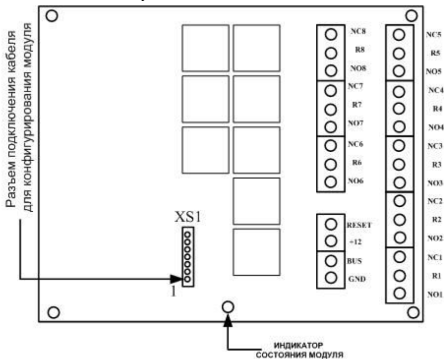
Рисунок 1 Внешний вид платы модуля
