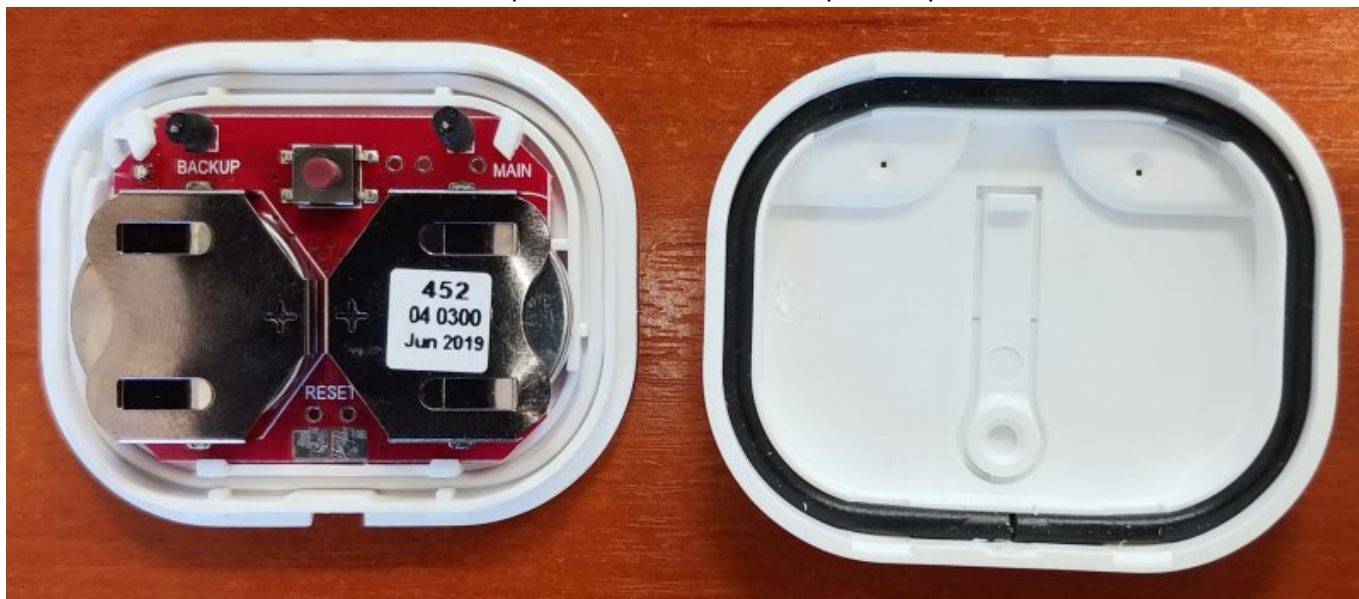
Рисунок 1. Извещатель с открытой крышкой
