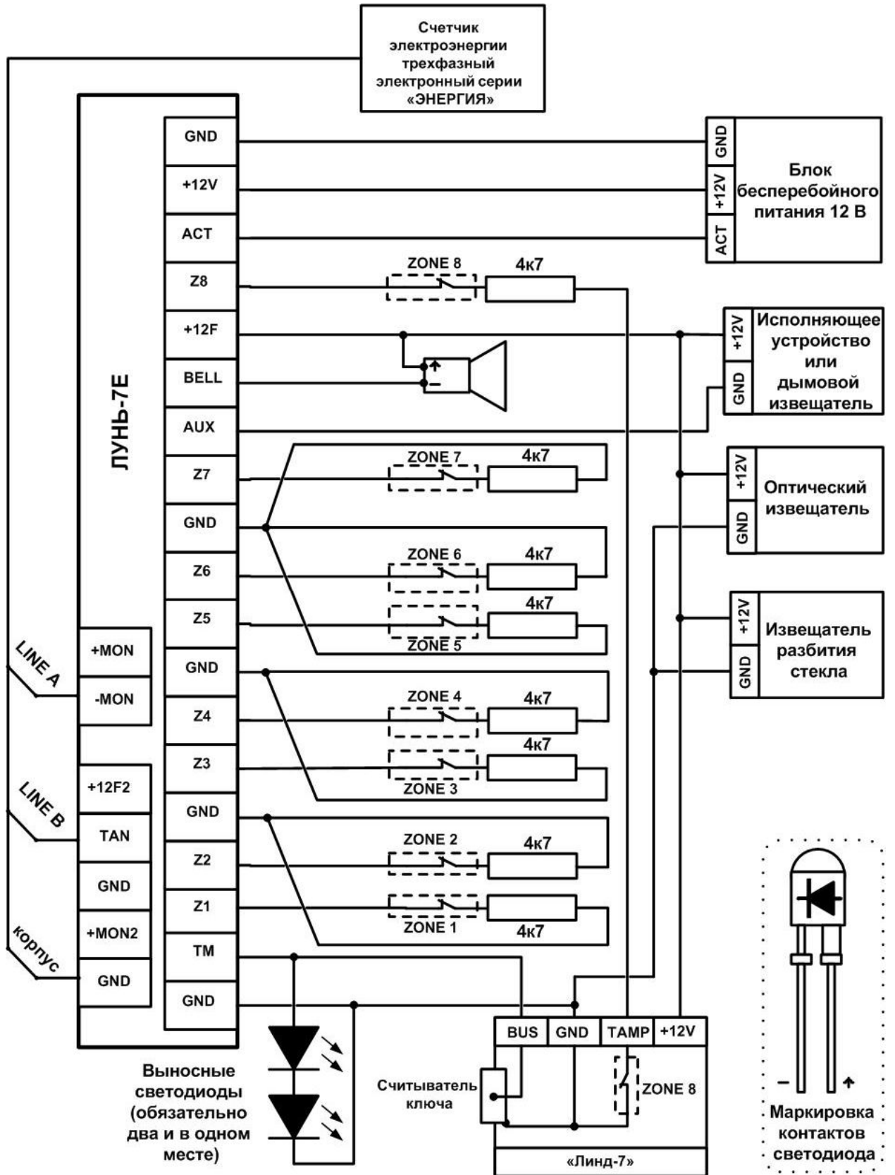
Рисунок 2 Схема подключения внешних устройств и извещателей (пример)
