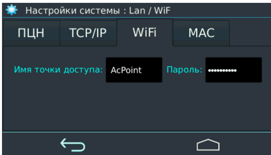
Рисунок 25. Настройки WiFi
