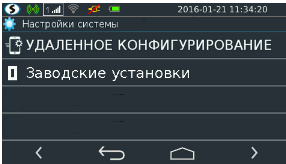
Рисунок 4. Системные настройки (4)
