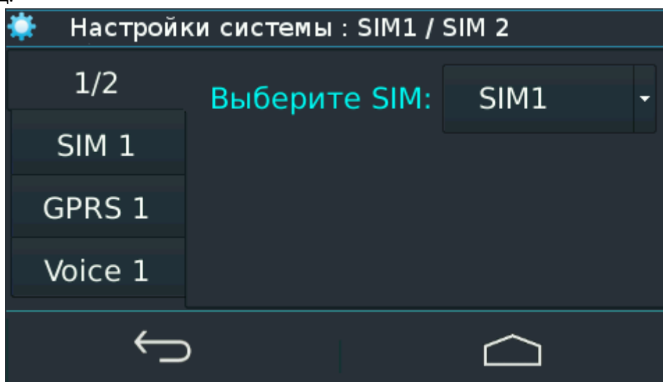
Рисунок 14. Настройки SIM (1)
