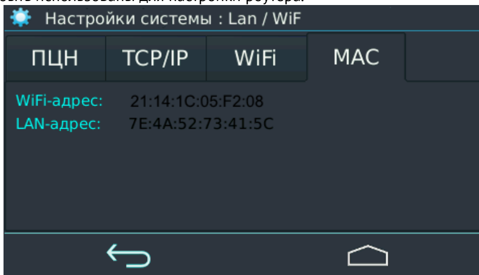
Рисунок 26. MAC-адреса ППКОП
