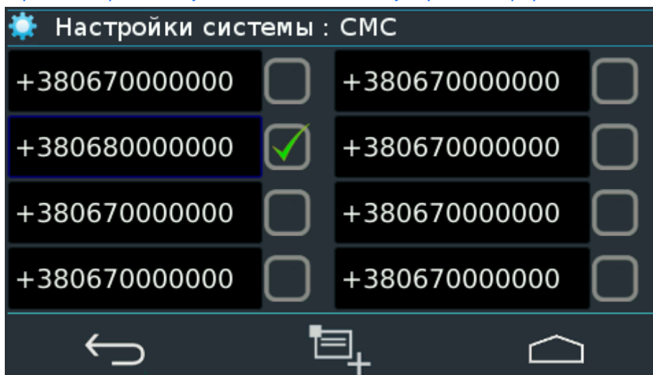
Рисунок 35. Настройки SMS
