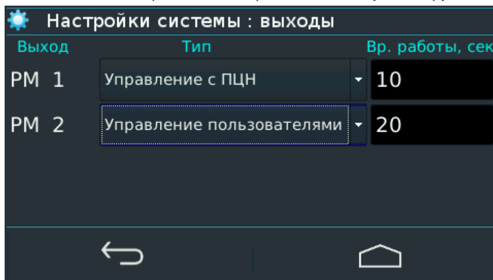
Рисунок 27. Настройка выходов
