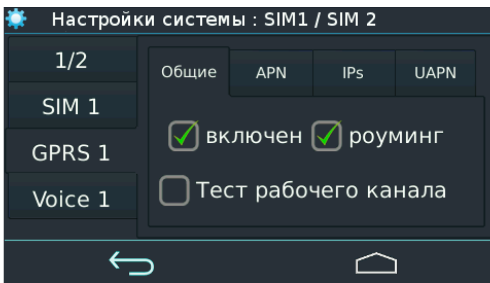
Рисунок 16. Включение GPRS
