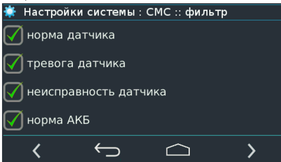
Рисунок 36: Фильтр сообщений
