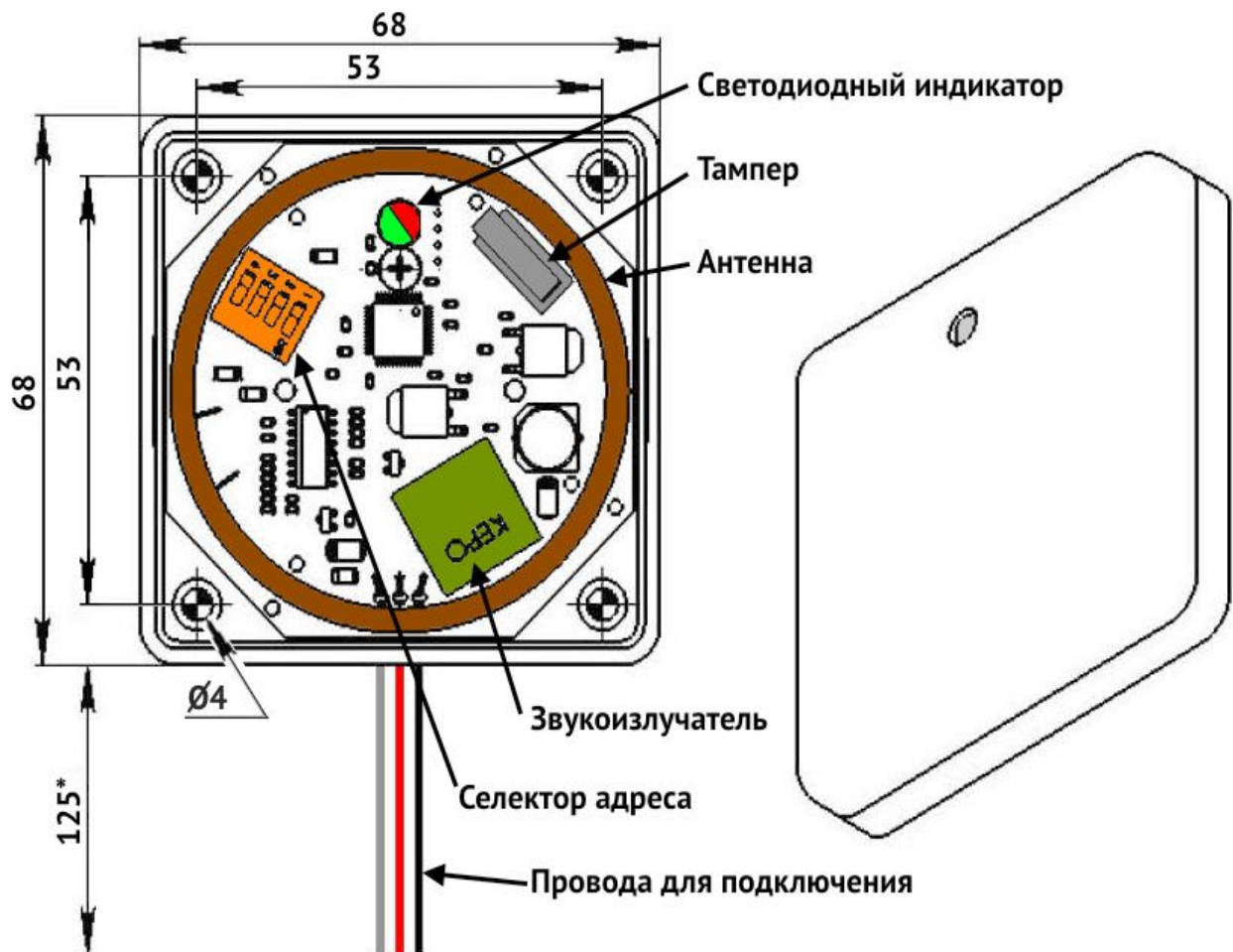
Рисунок 1. Считыватель «Линд-ЕМ»
