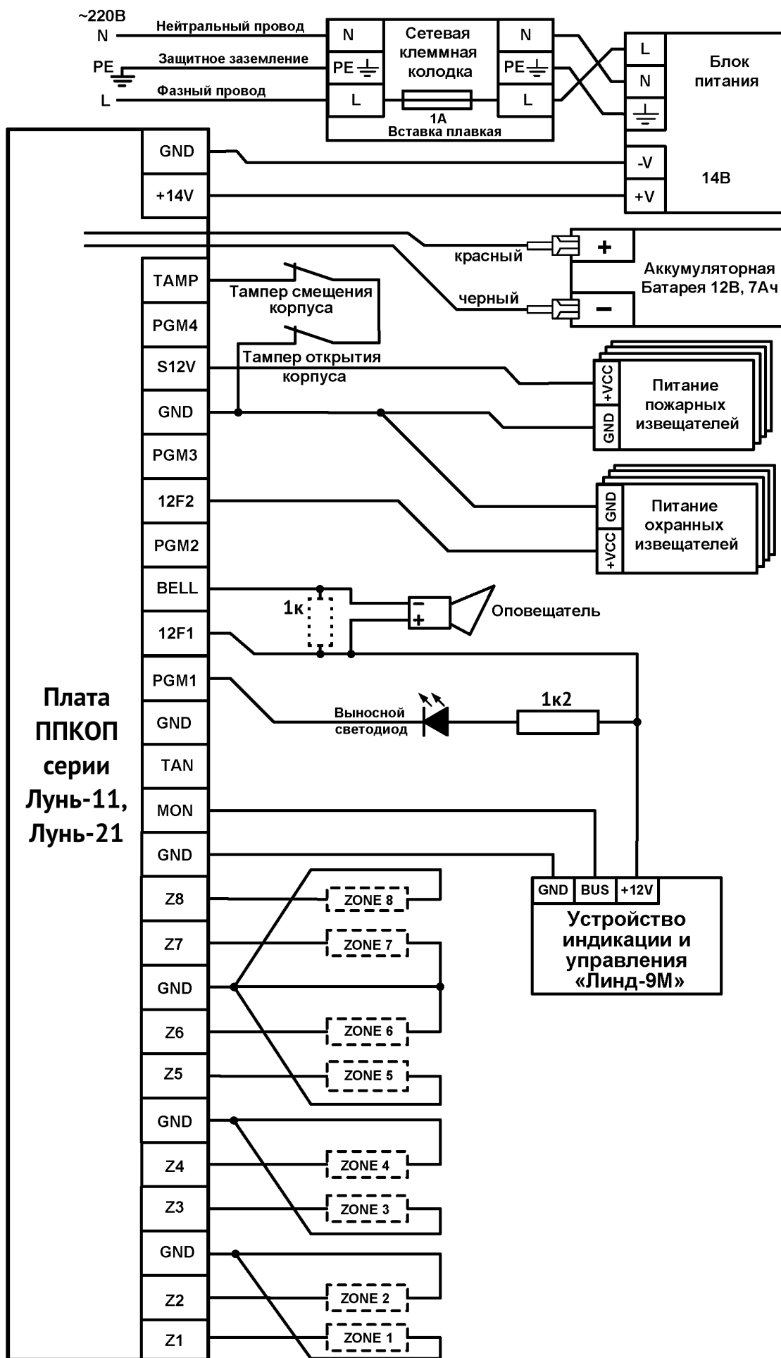
Рисунок 3. Схема подключения УИУ
