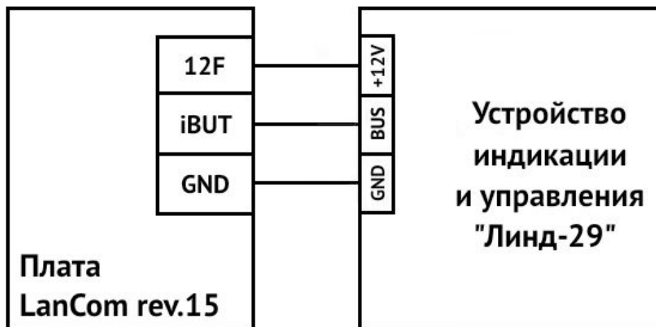
Рисунок 7. Схема подключения к устройству LanCom rev.15 в режиме «Без ППК»
