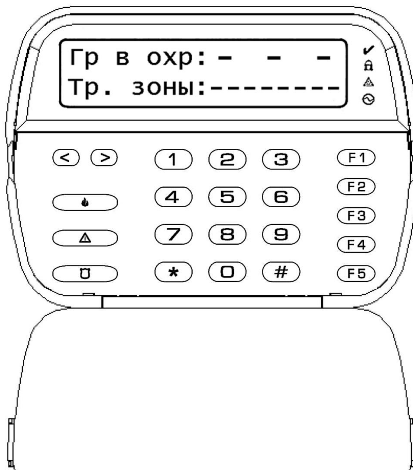
Рисунок 1. Устройство индикации и управления «Линд-10». Вид спереди с открытой крышкой.
