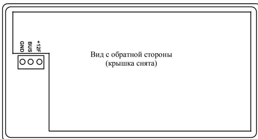
Рисунок 6 Устройство индикации и управления «Линд-Т»
