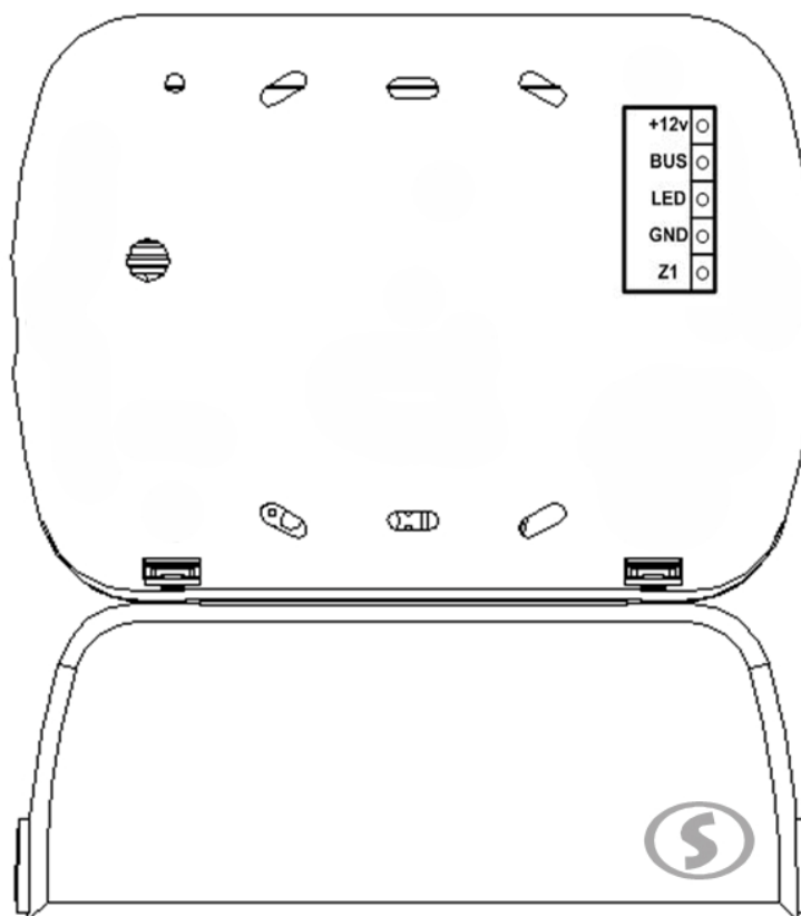
Рисунок 10. Устройство индикации и управления «Линд-10». Вид сзади.
