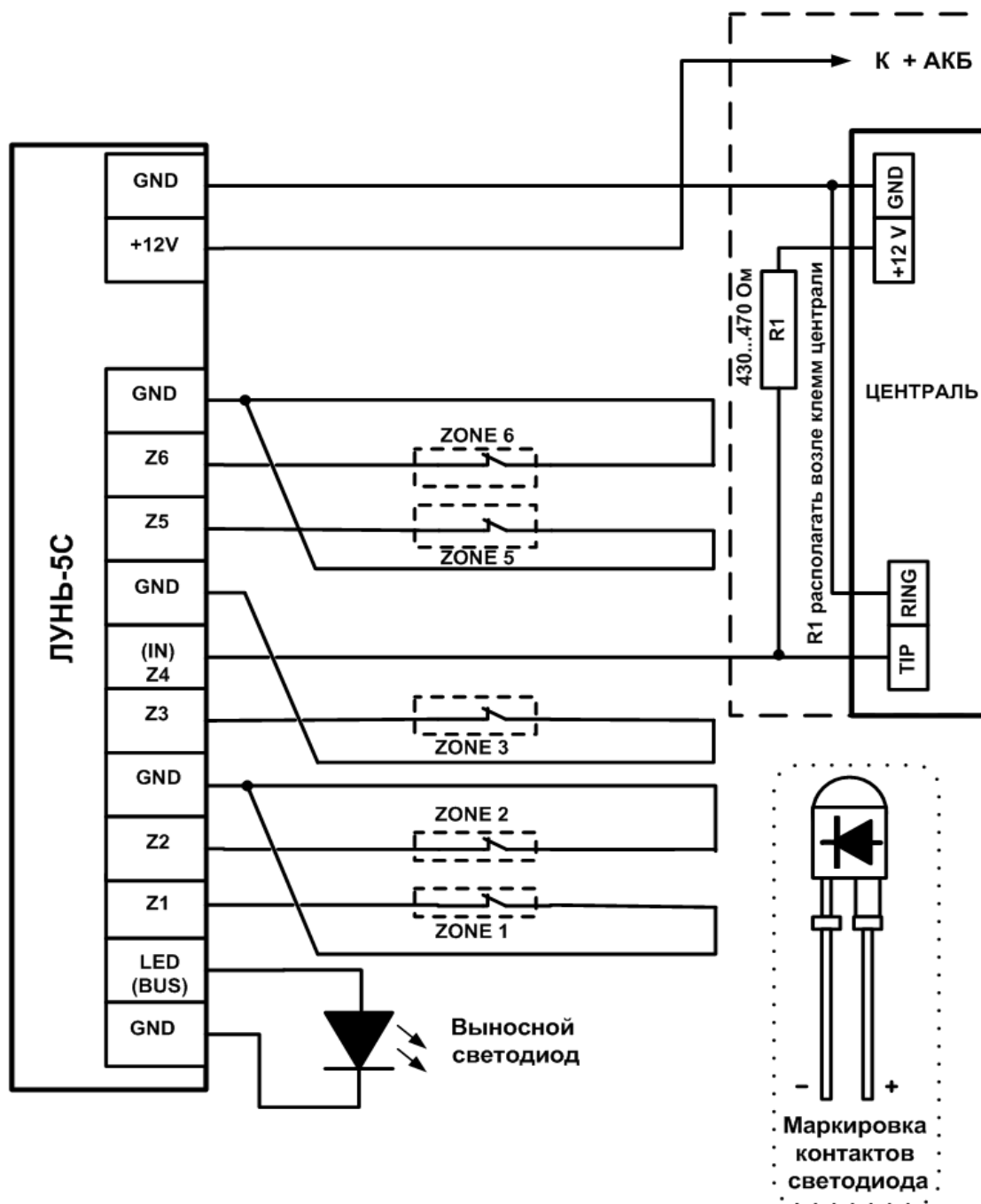
Рисунок 2 Схема подключения ОУС «Лунь-5С» к охранному прибору (централю).
